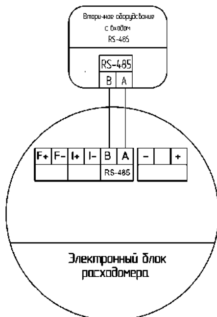
Рисунок 5.18 – Схема подключения электронного блока по интерфейсу RS-485
