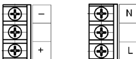
Рисунок 5.5 Наклейка усилителя генераторной катушки с питанием от источника постоянного тока (слева) и переменного тока (справа)
