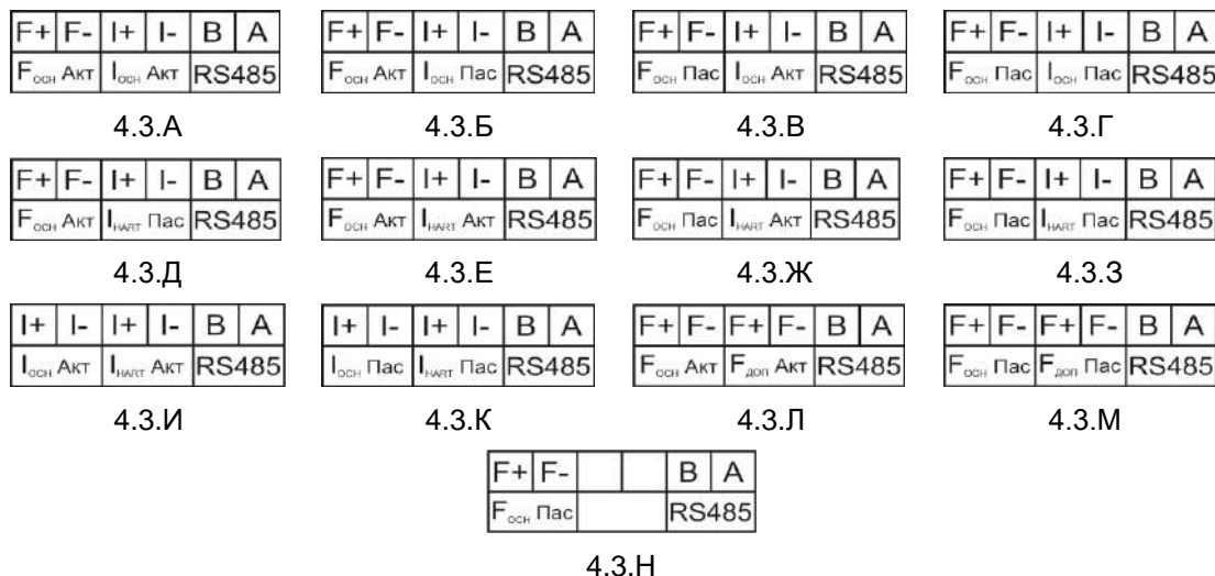
Рисунок 4.3 - Виды наклеек выходных сигналов
